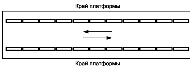
Рисунок А.4 - Форма рифления - одноэлементная тактильная полоса с плоской вершиной (шугцлия), используемая для обустройства протяженных предупреждающих ТНУ вдоль края платформ различного назначения
